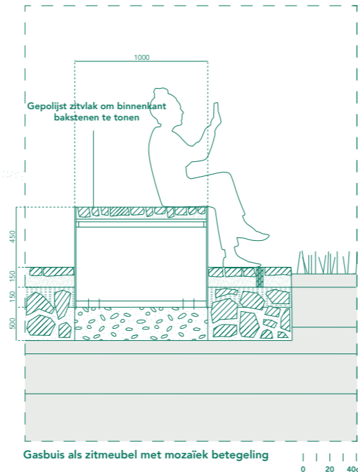
Drasn. E: Gaserfpad, gradaties aan verharding
