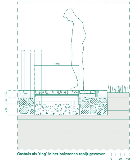
Drasn. D: Gaserfpad met gasbuis
